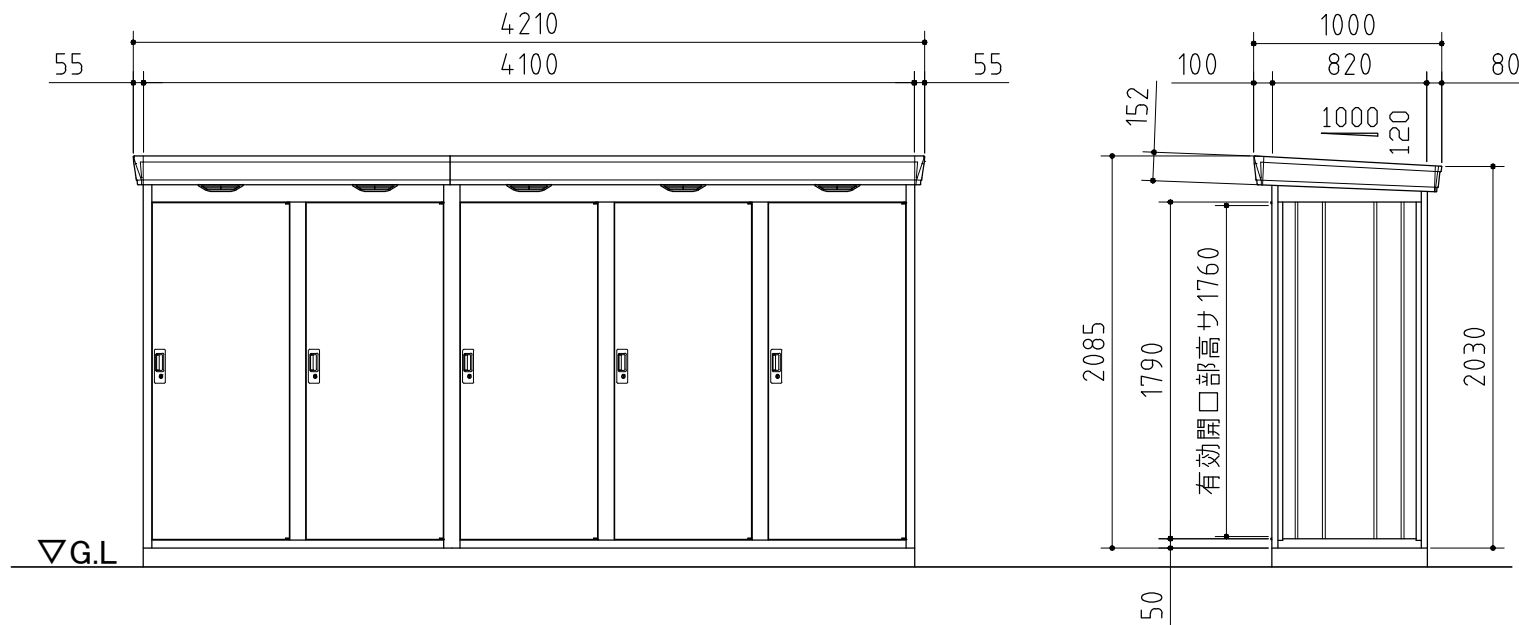
正面図
